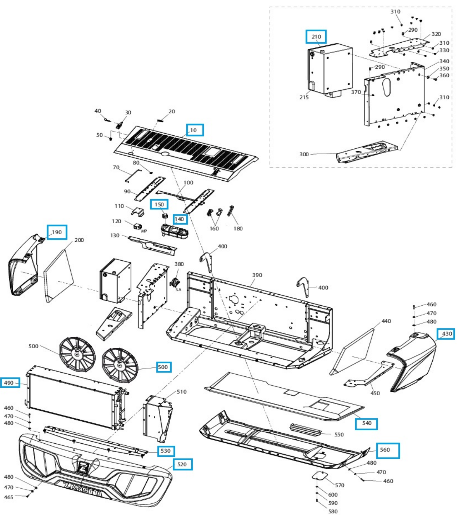
Tav.1007
